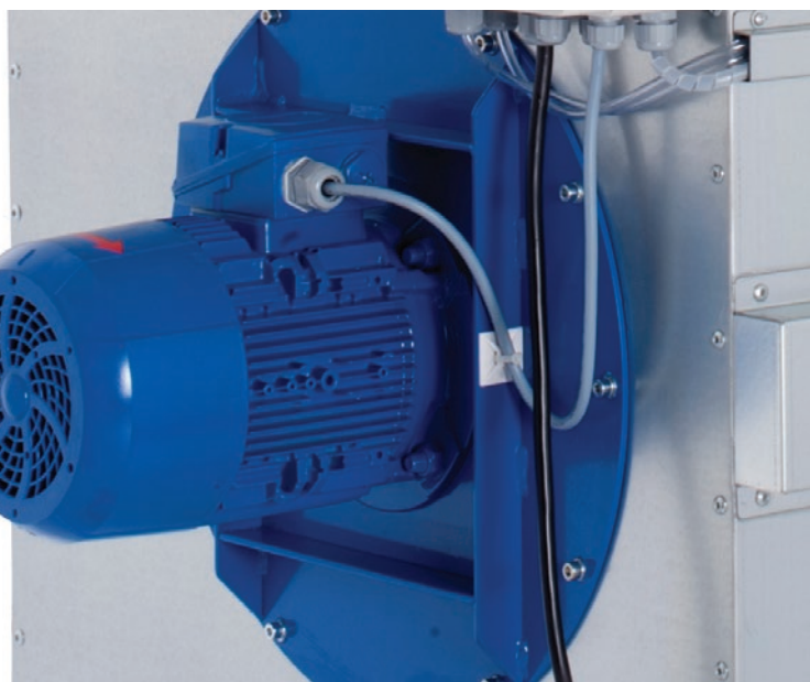
Ilustracja górna: Vacumobil VT 200 z silnikiem energooszczędnym 4,0 kW (IE3)
